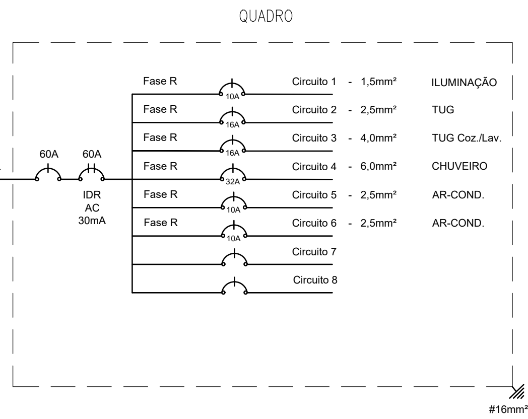
3 DIAGRAMA UNIFILAR SEM ESCALA
